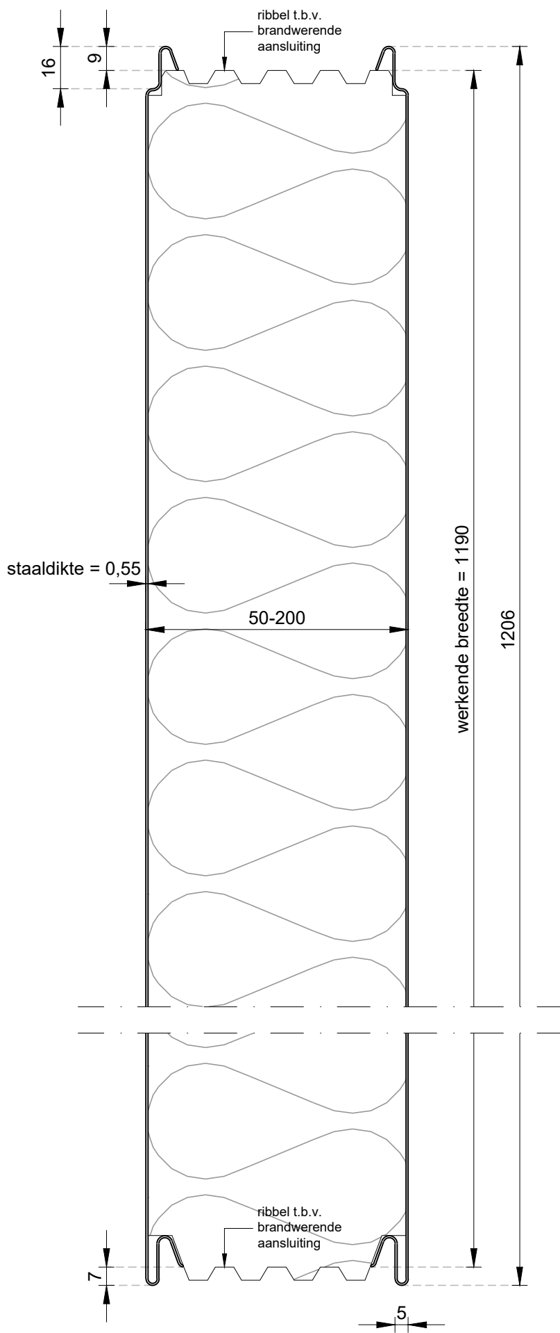
Doorsnede steenwol paneel
