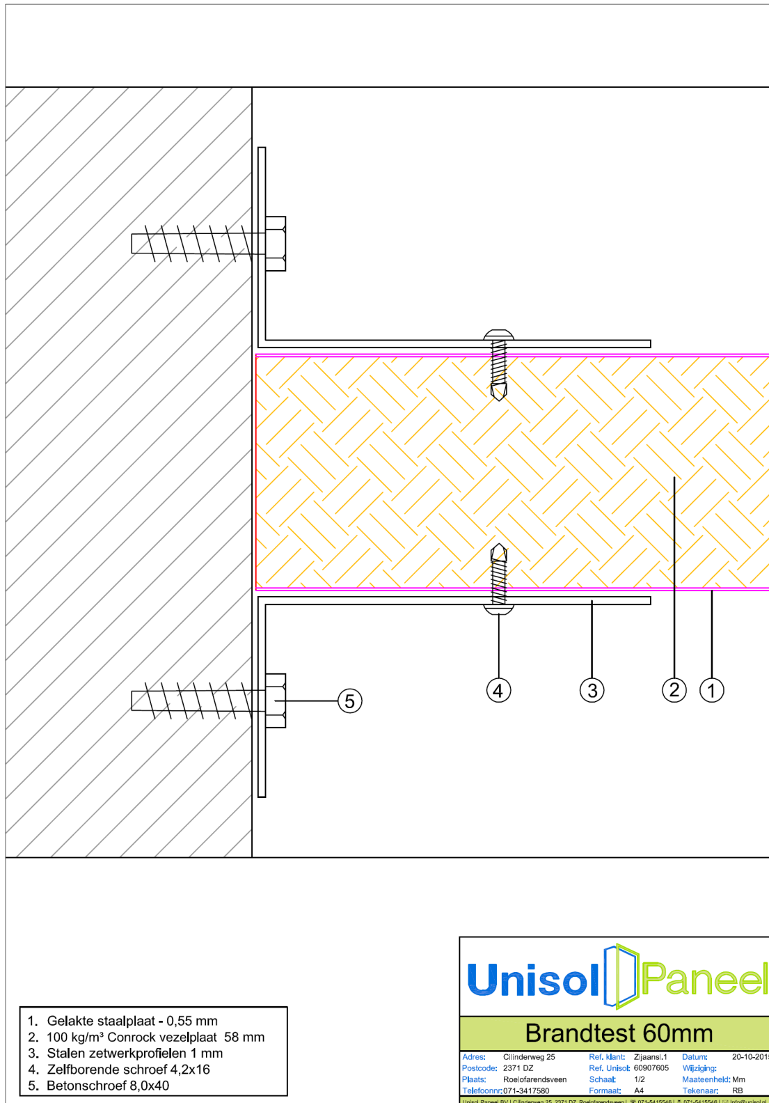
Figuur 5: vaste verticale aansluiting
