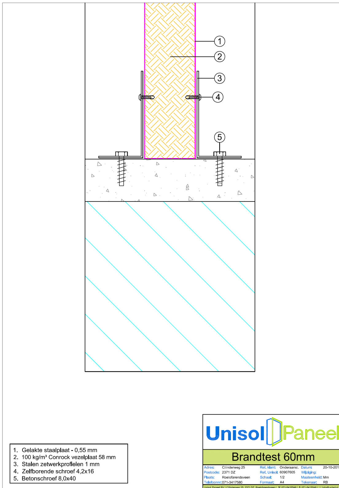
Figuur 4: onderaansluiting
