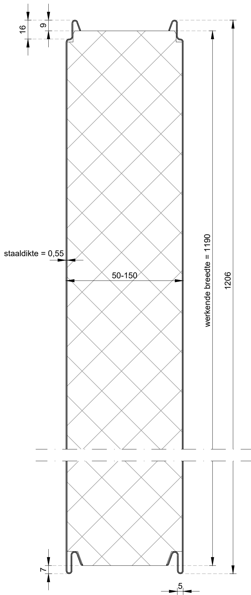
Doorsnede PIR paneel
