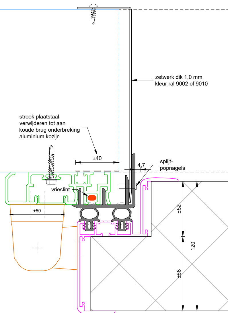
Detail, scharnierzijde schaal 1:2
