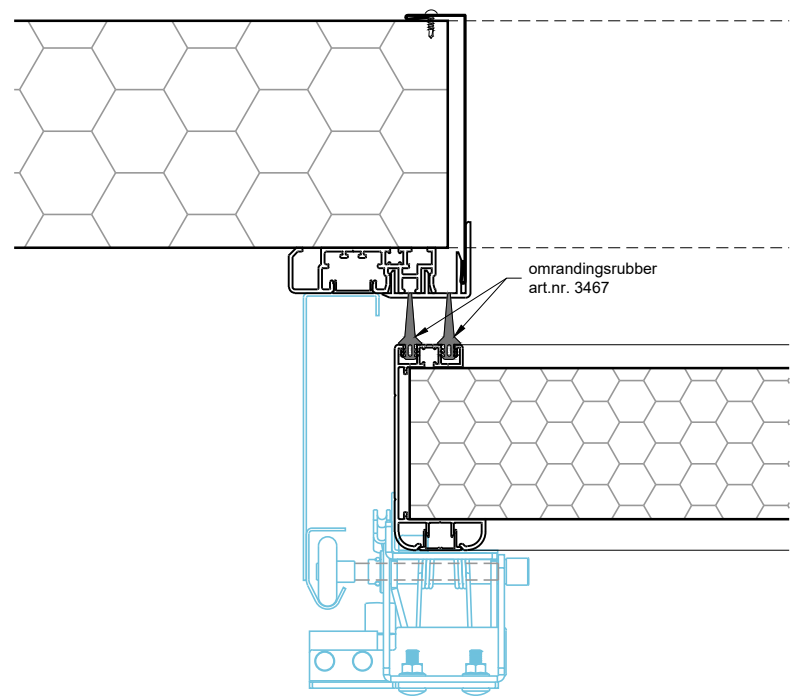
Detail 4 (koel-/vriescel uitvoering)
