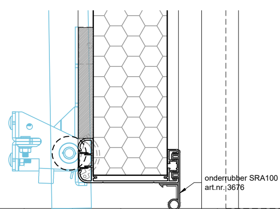
Detail 1a (koelcel uitvoering)
