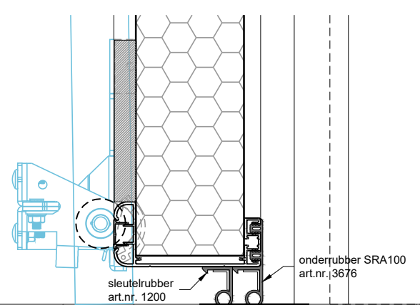
Detail 1b (vriescel uitvoering)
