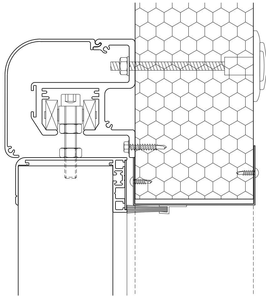
Detail 02 schaal 1:2
