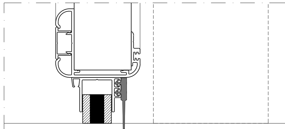
Detail 01 schaal 1:2
