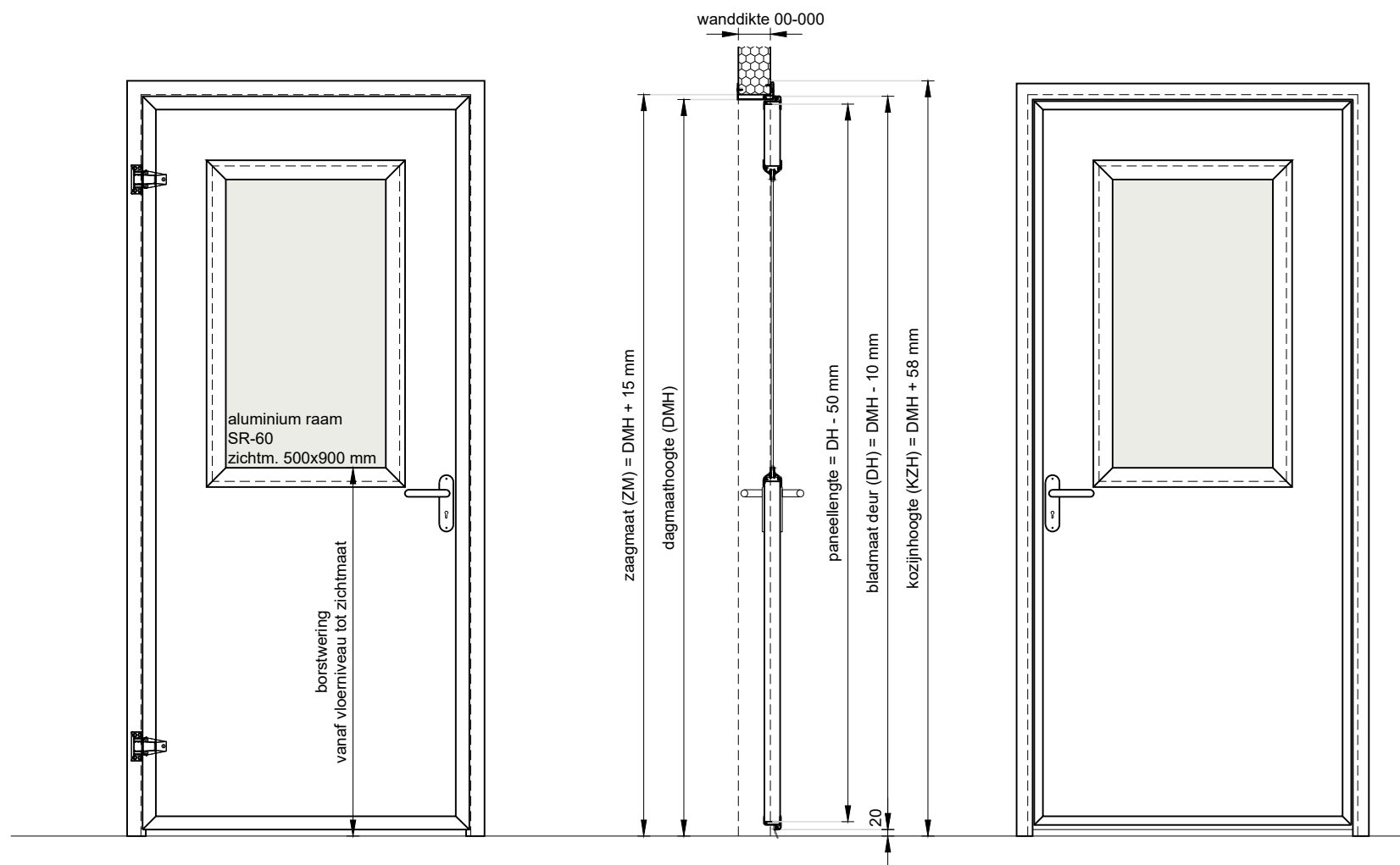
Vooraanzicht schaal 1:20
